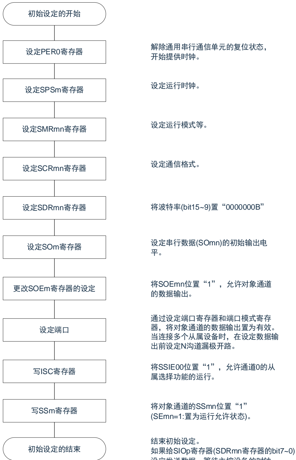
图12-88从属发送和接收的初始设置步骤
