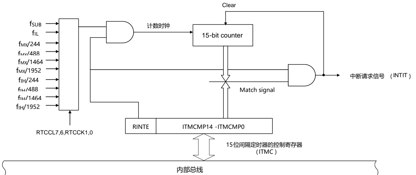
图7-1 15位间隔定时器的框图
