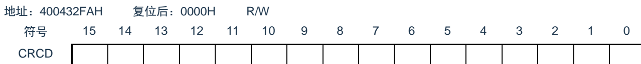
图22-5 CRC数据寄存器 (CRCD) 的格式
