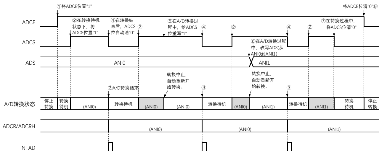
图10-21 软件触发模式（选择模式、单次转换模式）的运行时序例子
