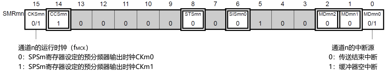
图12-87从属选择输入功能 (SSPI00) 从属发送和接收时的寄存器设置内容例子(1/2)
