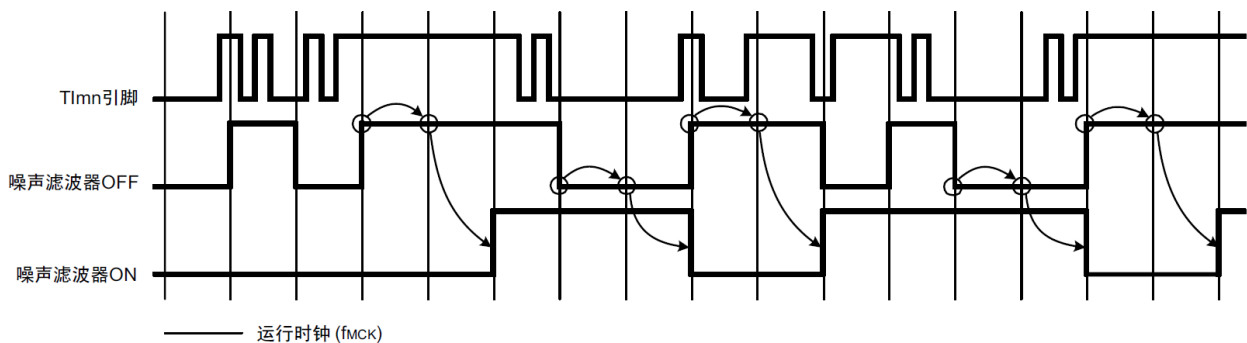
图 5-41：Tlmn输入引脚在噪声滤波器ON或者OFF情况下的采样波形
