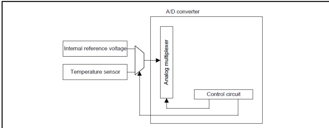
图 23-1温度传感器框图
