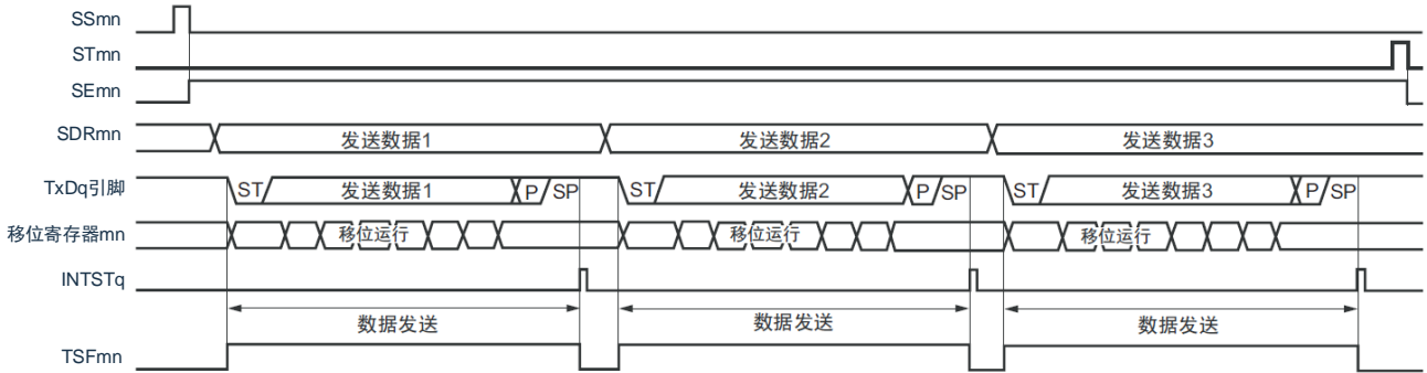
图12-101 UART发送（单次发送模式）的时序图
