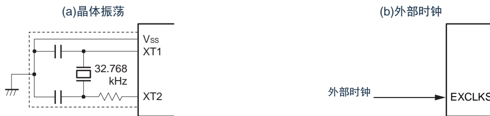
图4-14 XT1振荡电路的外接电路例子
