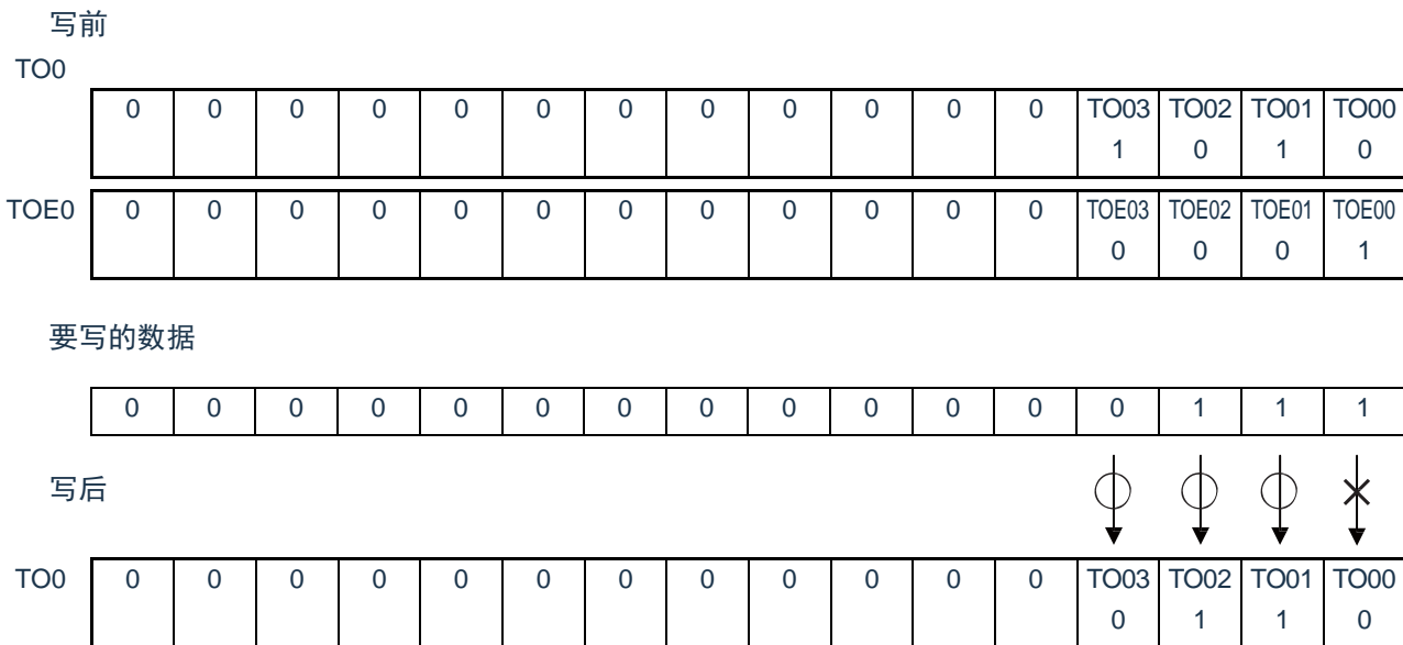
图 5-37: TO0n位的一次性操作例子
